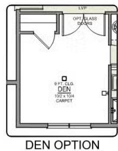
DEN OPTION
